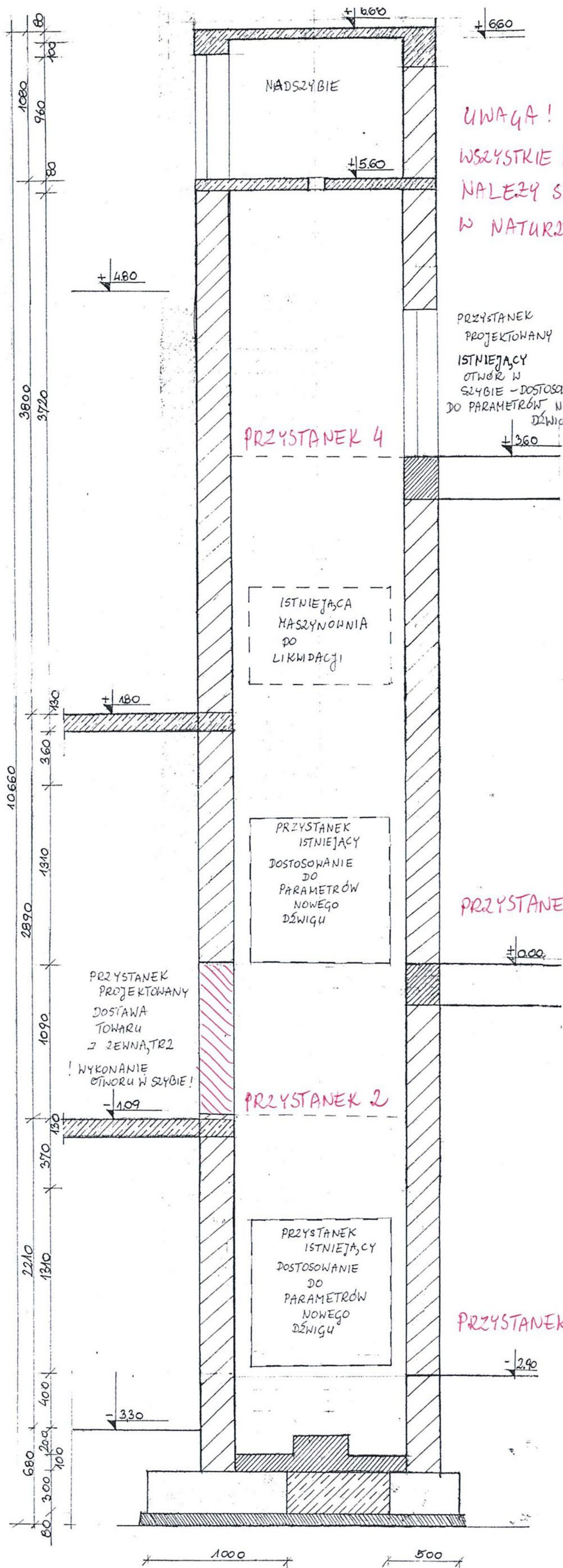
PRZEKRÓJ A-A
